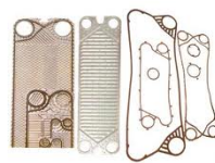
Plokštelės ir sandarikliai su apvalkalu
